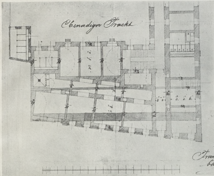
30. A dunaparti szárny tervrajza. Földszint.
