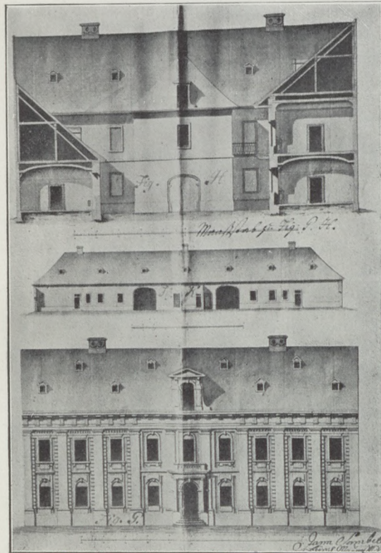
22. Sambelli János terve a pesti nemzeti iskola építésére (1799).
