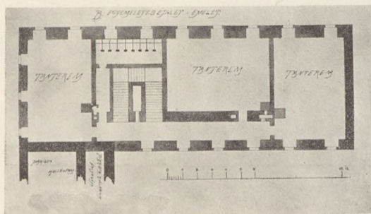
20. Jung József terve a pesti nemzeti iskola építésére.
