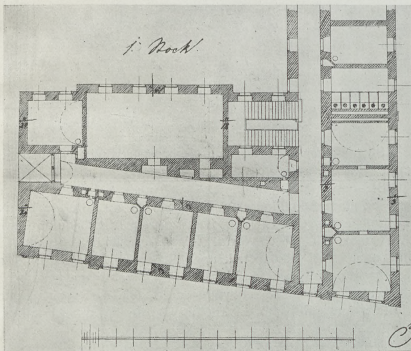
31. A dunaparti szárny tervrajza. Első emelet
