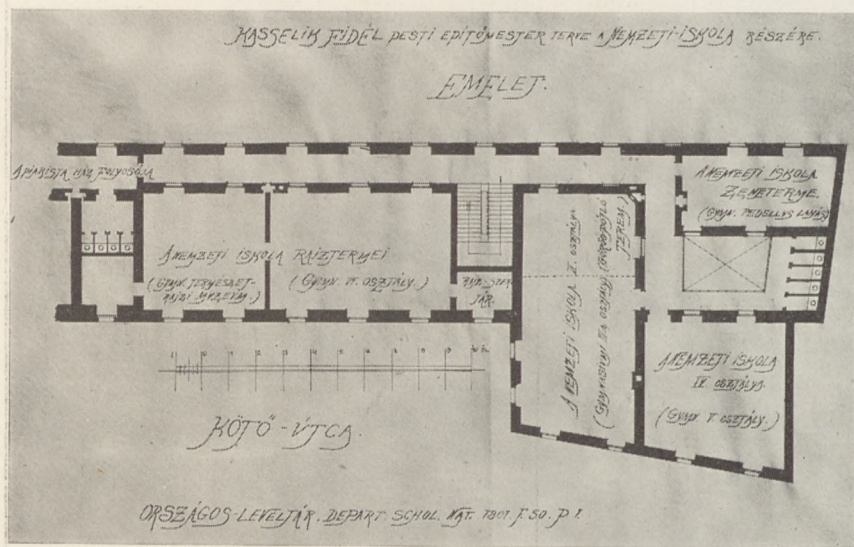
23. A kötő-utcai nemzeti iskola tervrajza. Emelet.
