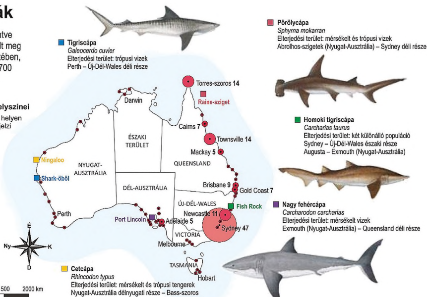
Cápa-fajok, cápa-zónák és cápatámadások Ausztrália partjainál [1]
