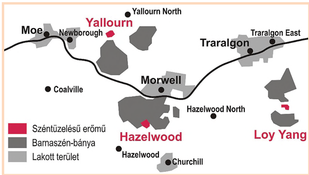
Széntelepek Victóriában (sötétszürkével) és a szénrel fűtött erőművek (pirossal). Világosszürkével a lakott helyeket jelölték. 66
