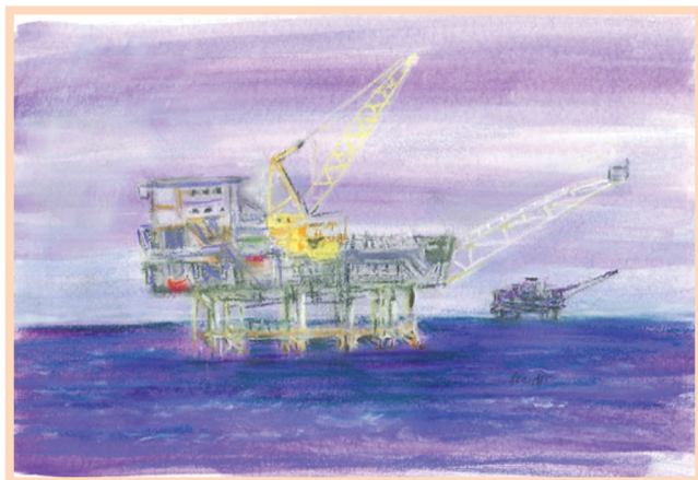
Az első tengeri kőolajkút Ausztráliában: az 1967-ben elkészült Kingfisher-platform a Bass-szorosban, Victoria állam keleti partjainál
