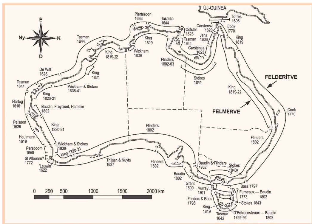
Feltérképezve és felmérve: tengeri expedíciók az ausztrál partok mentén 13
