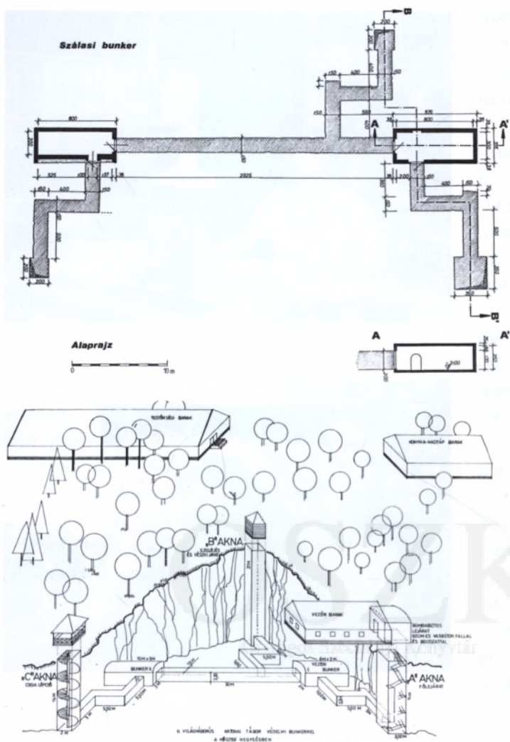
A kőszegi Szálasi-bunker alaprajza és az elképzelt rekonstrukció terve (H. Reinhoffer Éva munkája)
