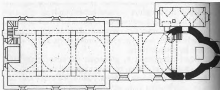
38. A hidegségi kerektemplom alaprajza
