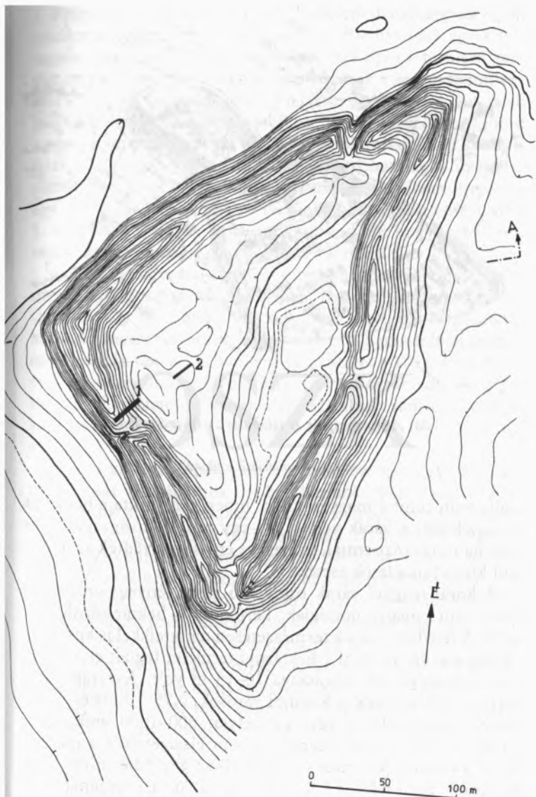
24. A szabolcsi földvár rétegvonalas helyszínrajza
