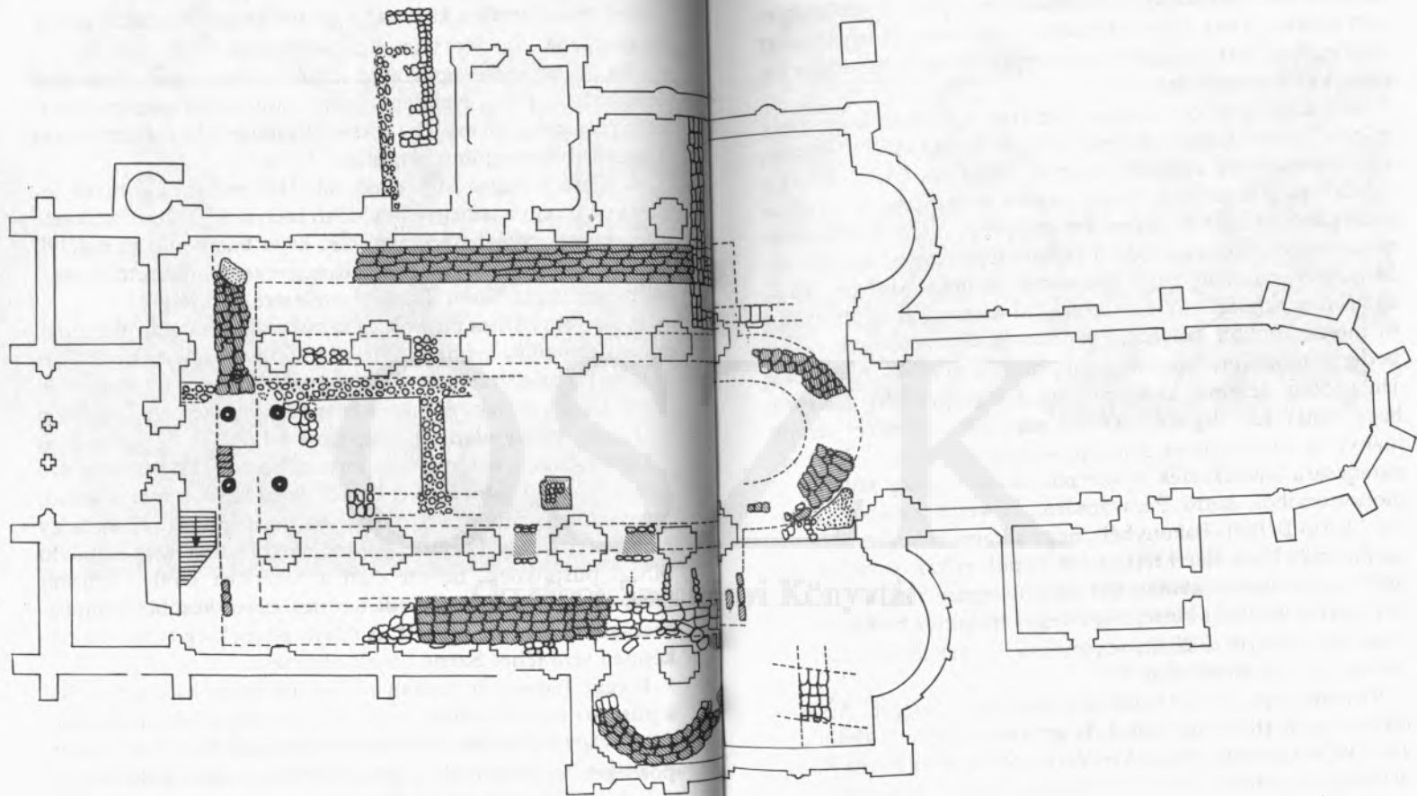
34. A gyulafehérvári székesegyház alaprajza
