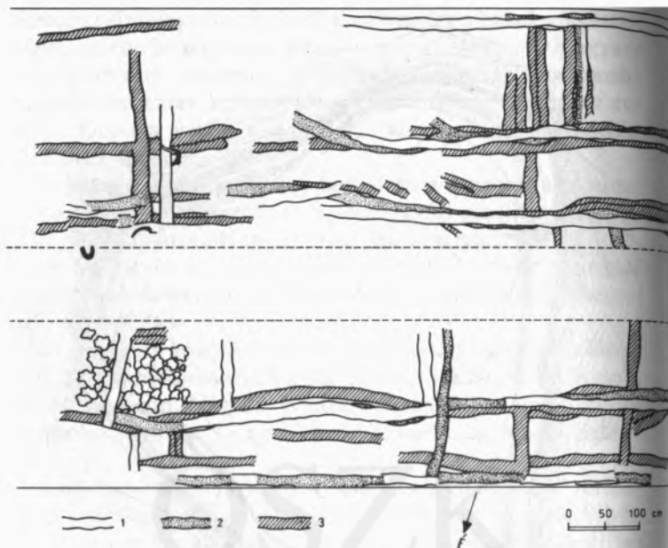
22. Jellegetes 10. századi sáncszerkezet
