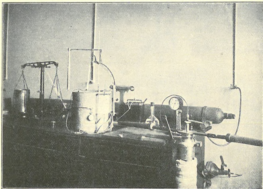
Vizkaloriméter
