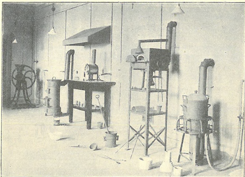
Gázolvasztó és hevítő kemenczék
