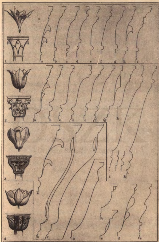
A NÉGY VELENCZEI VIRÁGOS OSZLOP-REND.
