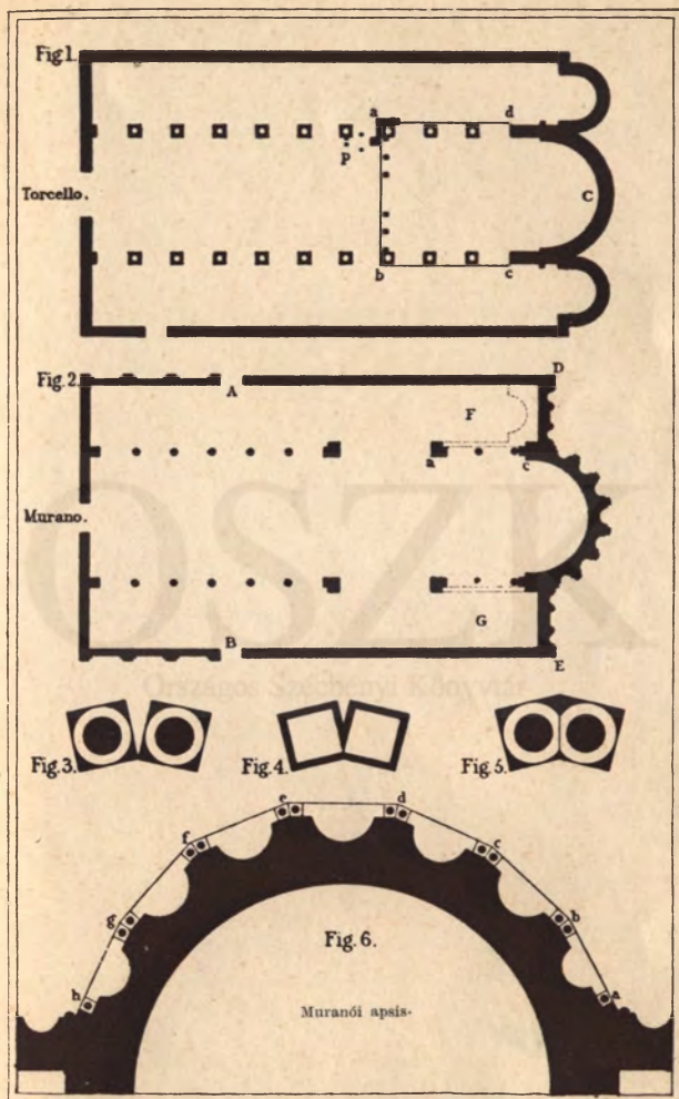
A TORCELLÓI ÉS MURANÓI BAZILIKÁK ALAPRAJZA.
