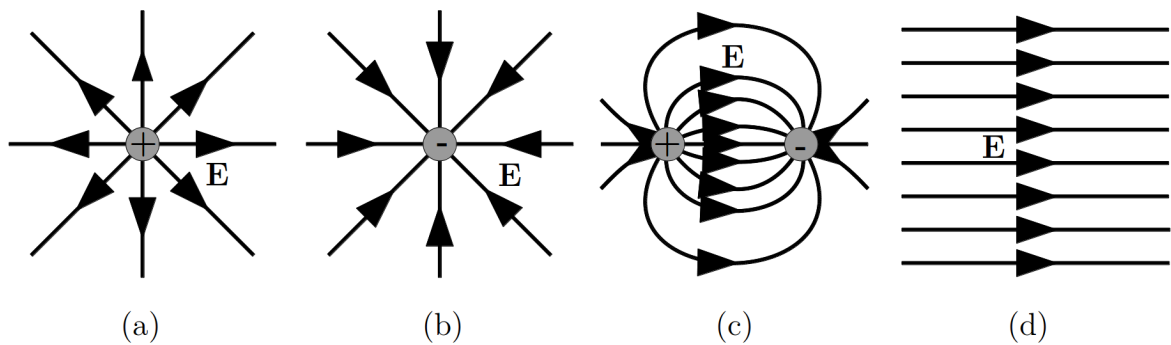
1.7. ábra. Az elektromos erőter szemléltetése erővonalakkal
