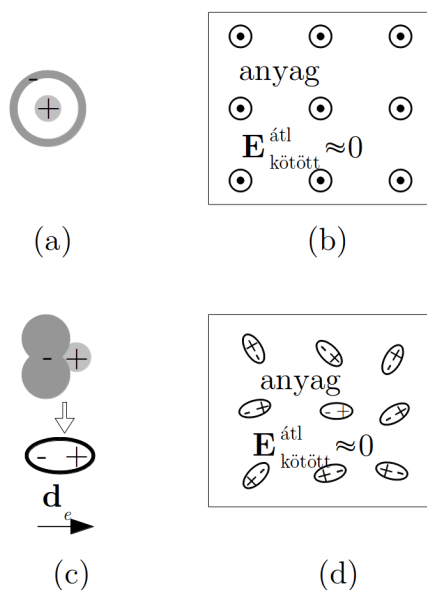
2.1. ábra. Gömbszimmetrikus töltéseloszlású (apoláros) (a.) és a pozitív és negatív töltés súlypontjában eltérő (poláros) molekula (c.) és a belőlük álló anyag (b. illetve d.) külső elektromos tér nélkül
