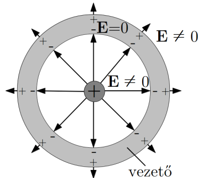
1.29. ábra. Üreges vezető belsejében elhelyezett töltés tere
