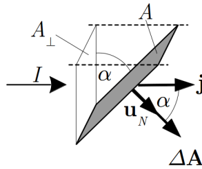
3.5. ábra. Az áramerősség számítása egy kis felületelem esetén
