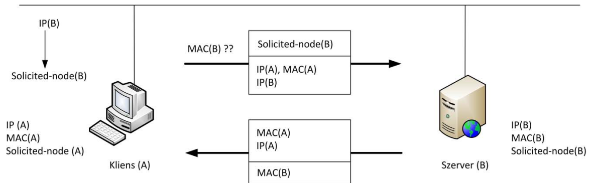
4.57. ÁBRA MŰKÖDÉSSEN A SOLICITED NODE CÍMZÉS
