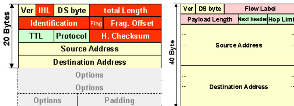
4.52. ÁBRA IPCSOMAGOK FEJLÉCEINEK ÖSSZEHASONLÍTÁSA
