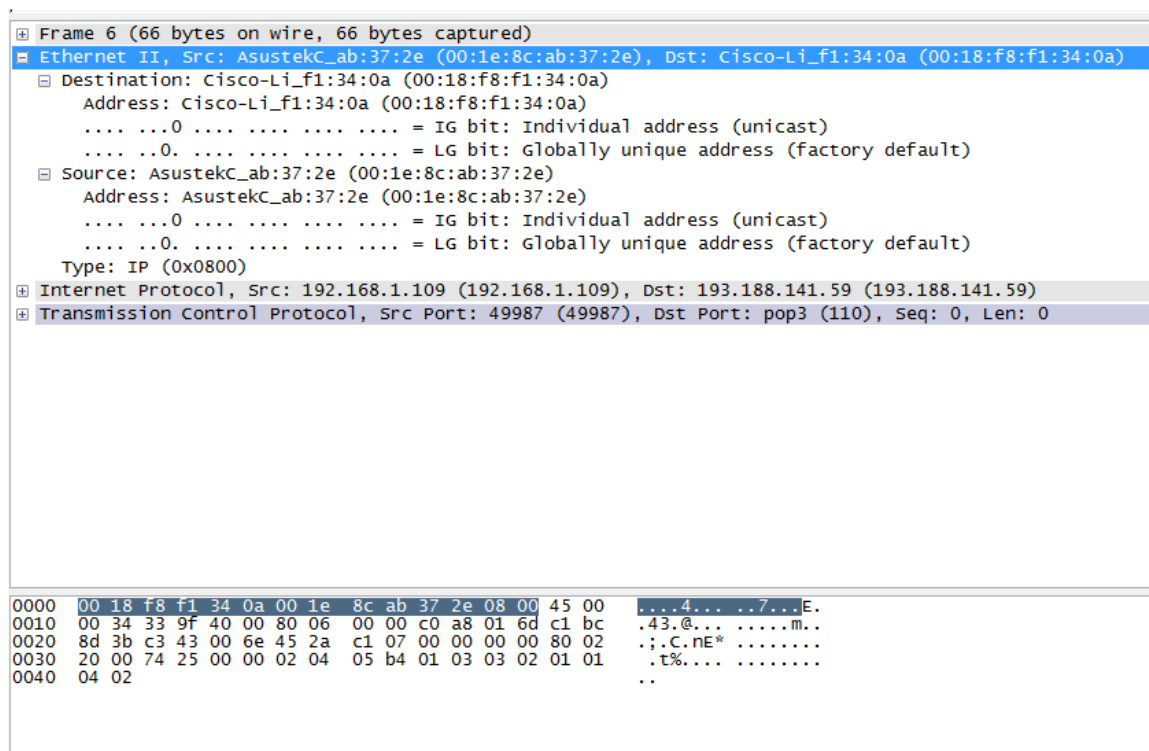
3.2. ÁBRA EGY ETHERNET II FRAME
