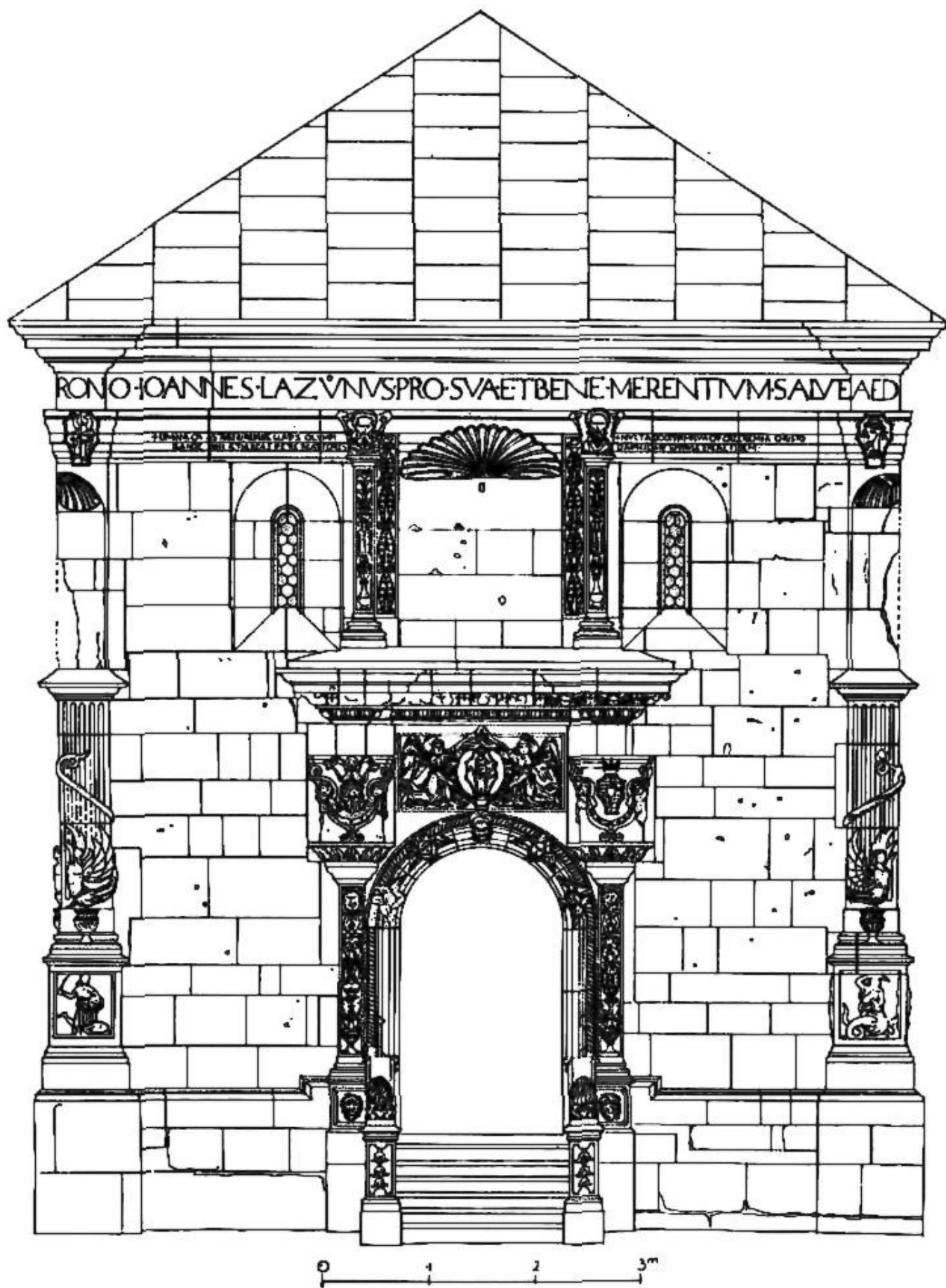
16. kép. A Lászay-kápolna északi homlokzata (Lux Géza)
