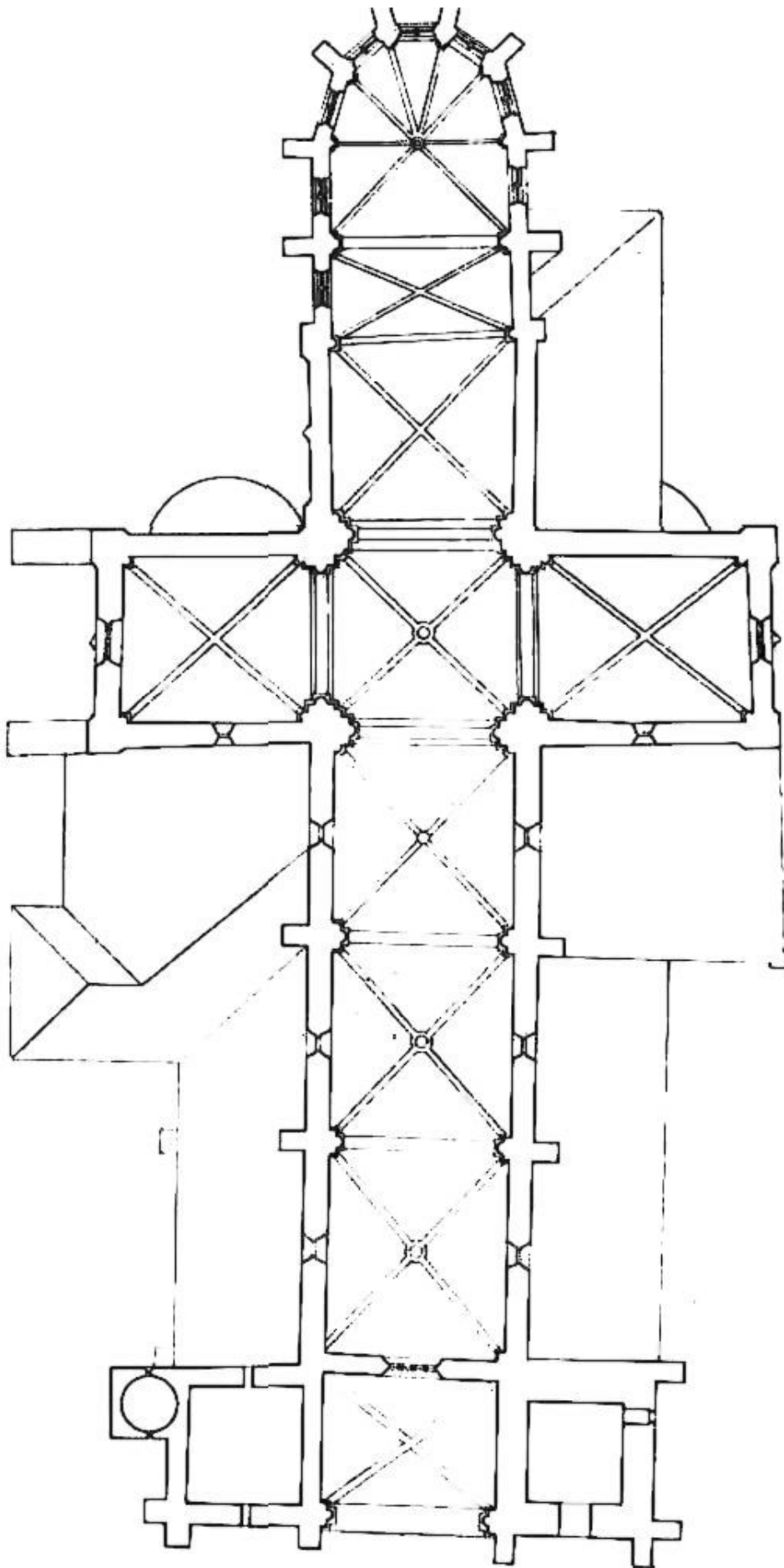
9. kép. A székesegyház emeleti alaprajza (Lux Géza)
