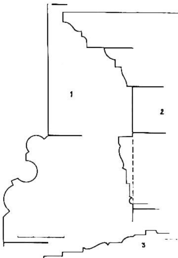
17. kép. 1. A székessygyház eredeti külső lábzatának metszete. 2. A Lászay-kápolna főpárkányának metszete. 3. A kápolna belső ajtajának metszete (Csányi Károly)
