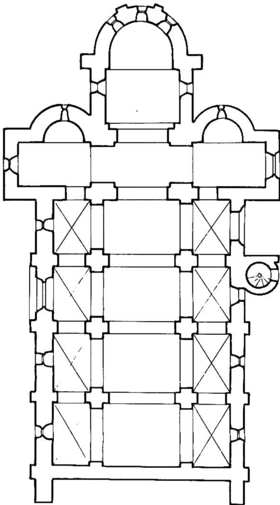
59. kép. Háromhajós bazilika alaprajza Uchiyben
