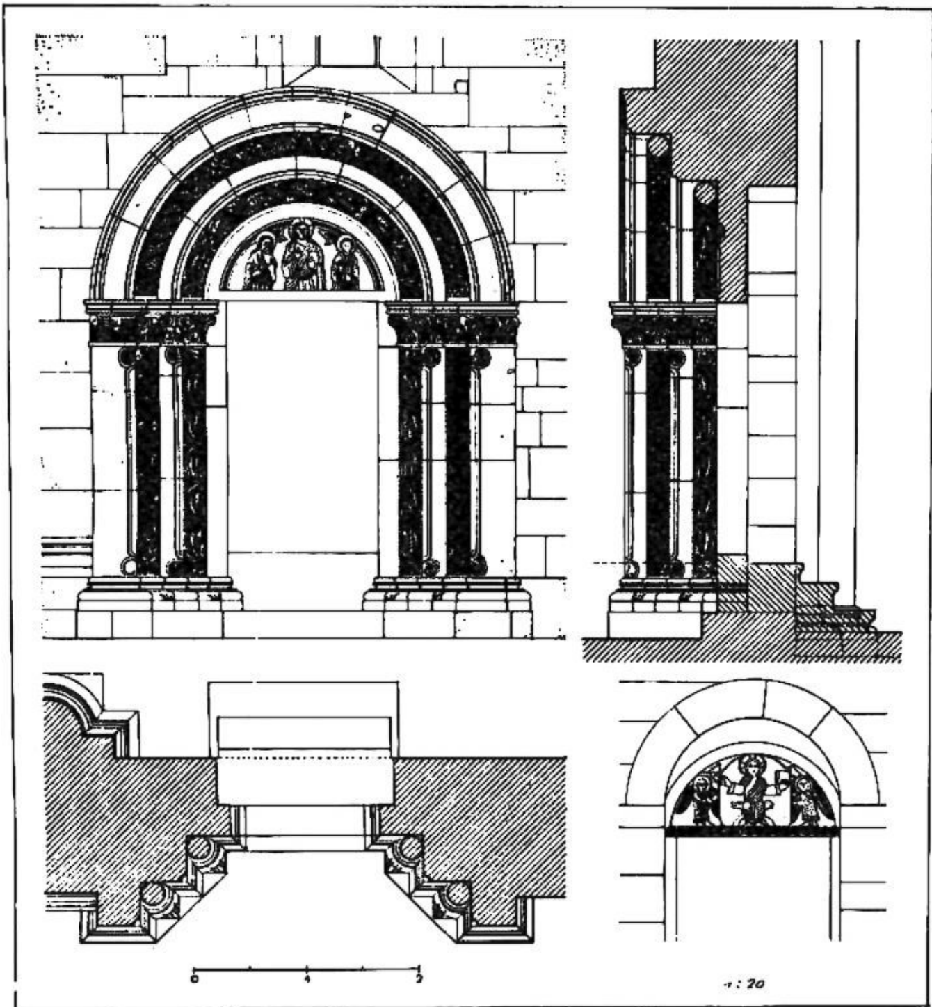
7. kép. A déli kapu nézete, metszete és alaprajza, valamint a XI. századi oronzatdombormű (Lux Géza)
