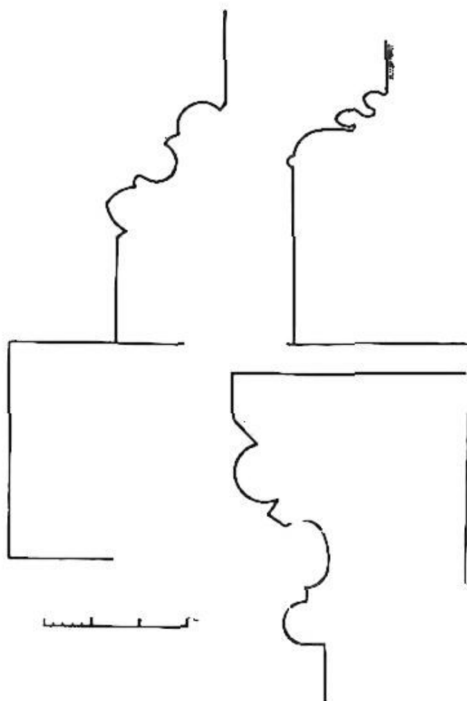
20. kép. 1—2. A nyugati kapubélett lábazonának metszetei. 3. A főhajó falpillér-fejlemezőnek metszete (Nagy Károly)
