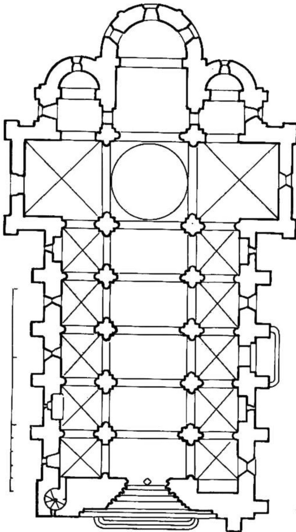
58. kép. A mauritiai háromhajós bazilika alaprajza
