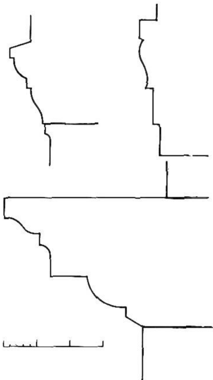
18. kép. A Lászay-kápolna nyugati, elfalazott ajtajának metszetei (Csányi Károly)
