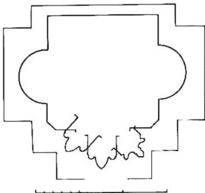
42. kép. Az északi mellékhajó 8. sz. pillérének bordaindítása (Möller István)
