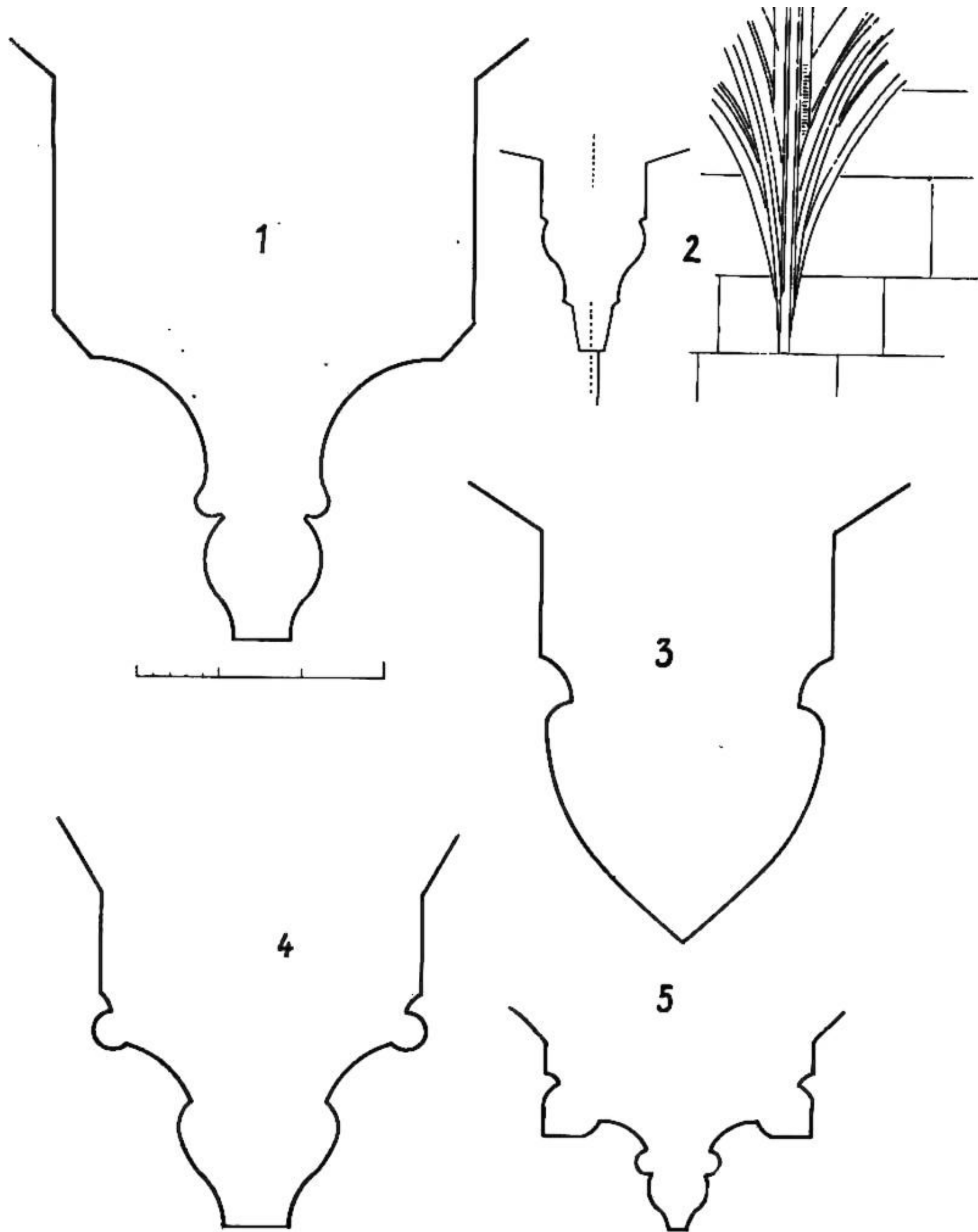
32. kép. Bordametszetek. 1. Várday-kápolna. 2. Lászy-kápolna. 3. Főszentély záródása. 4. Főhajó. 5. Mellékhajók nyugati boltszakaszai
