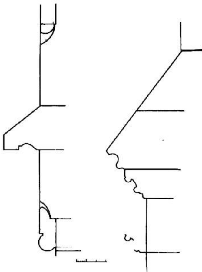
12. kép. A főszentély övpárkányának és a csanakatorony övpárkányának metszete (Csányi Károly)
