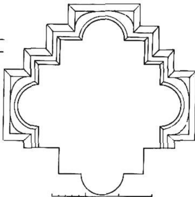
21. kép. A tizenkétosztású hajópillér alaprajza (Csányi Károly)
