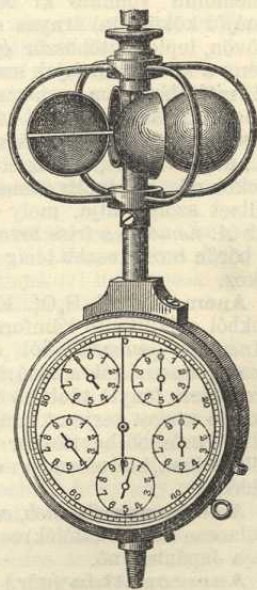
Robinson-féle anemométer.
