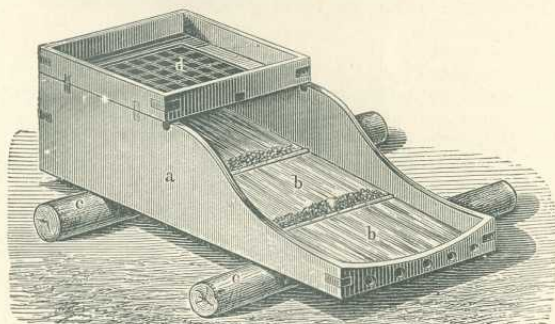
2. ábra. Aranymosó bölcös.
