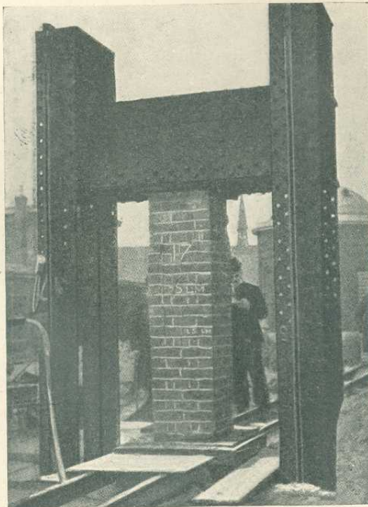
3. ábra. Teglapiiller törőpróbája.
