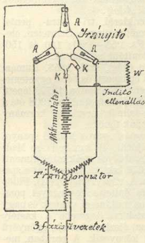
2. ábra. Higanygőz-irányító kapcsolása.
