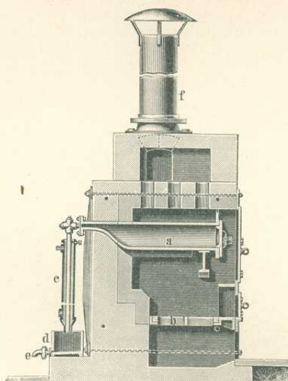
7. ábra. Fencsor-izzító retortás kemence.
