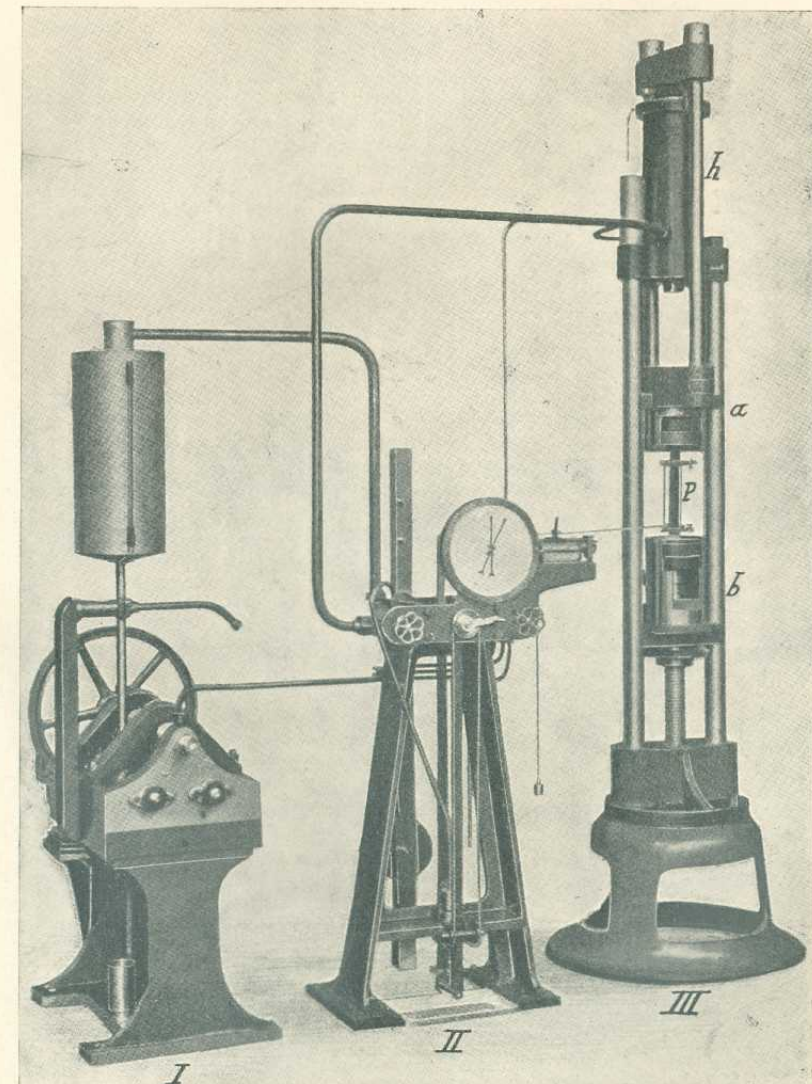
6. ábra. Szakító gép 20 tonna húzóerőig. (Amsler-Laffon.)
