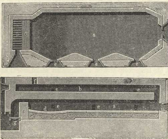
A tovalapátoló kemence függőleges és vízszintes metszete.
