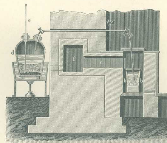
12. ábra. Klorizáló készülék.
