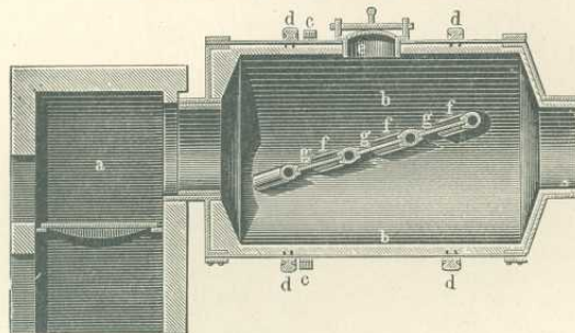
8. ábra. Brückner forgó kemencéje.
