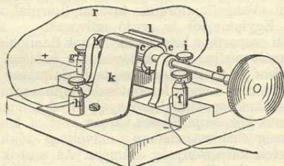
2. ábra. Ruhmkorff-féle áramfordító.
