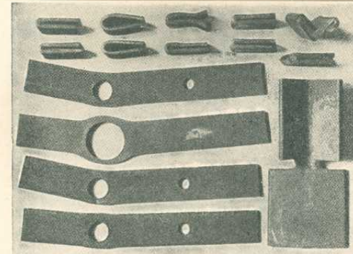
9. ábra. Vasvizsgálat (hajlító és egyéb technológiai próbák).
