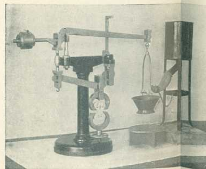
4. ábra. Szakító gép (cementvizsgálathoz).
