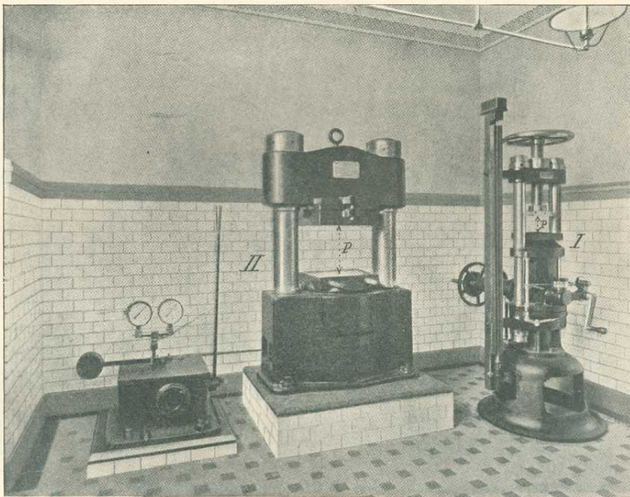
1. ábra. Cementsajtó (I); betonsajtó (II).
