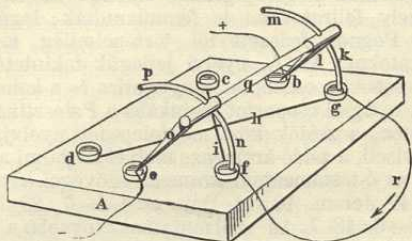
1. ábra. Pohl-féle áramfordító.
