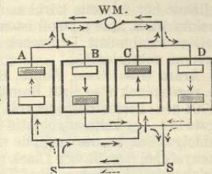
1. ábra. Áram útja az irányító cellában.
