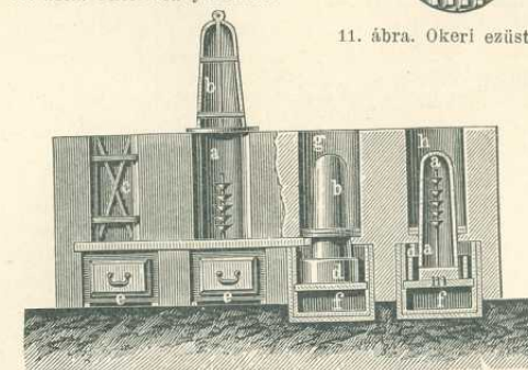
6. ábra. Fencsor-izzító kemence.
