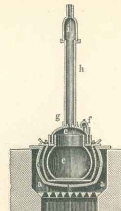
10. ábra. Okeri aranyfinomító.
