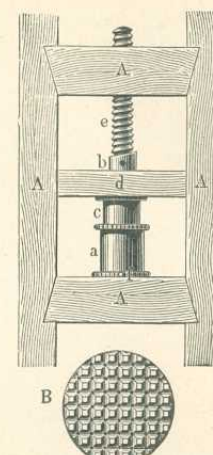
11. ábra. Okeri ezüstsajtó.
