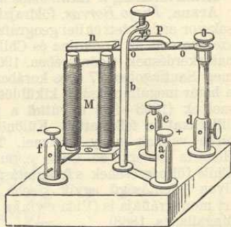
Wagner-féle kalapács.
