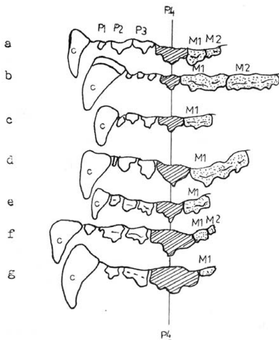
3. ábra. A felső előzáfogak és záfogak összehasonlítása néhány ragadozónál: a– Canis sp.; b– Ursus sp.; c– Martes sp.; d– Meles sp.; e– Herpestes sp.; f– Hyaena sp.; g– Felis sp. (M. Weber szerint, Dornescu&Nekrasovnál)
