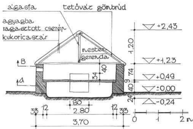
FÜGGŐLEGES METSZET
