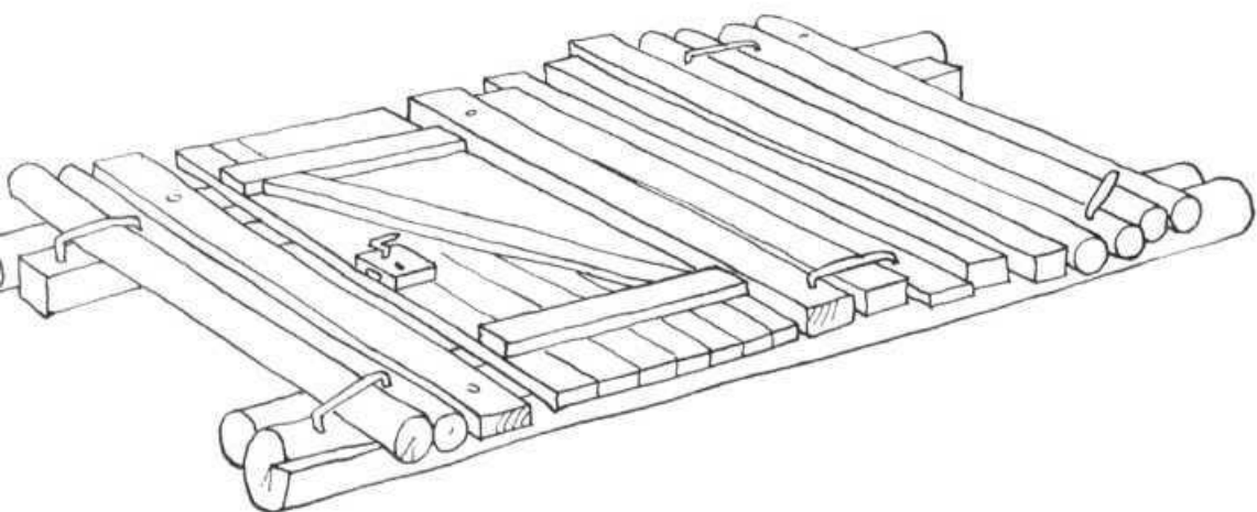
„LÁP”-nak nevezett szükségtutaj (rekonstrukció)
